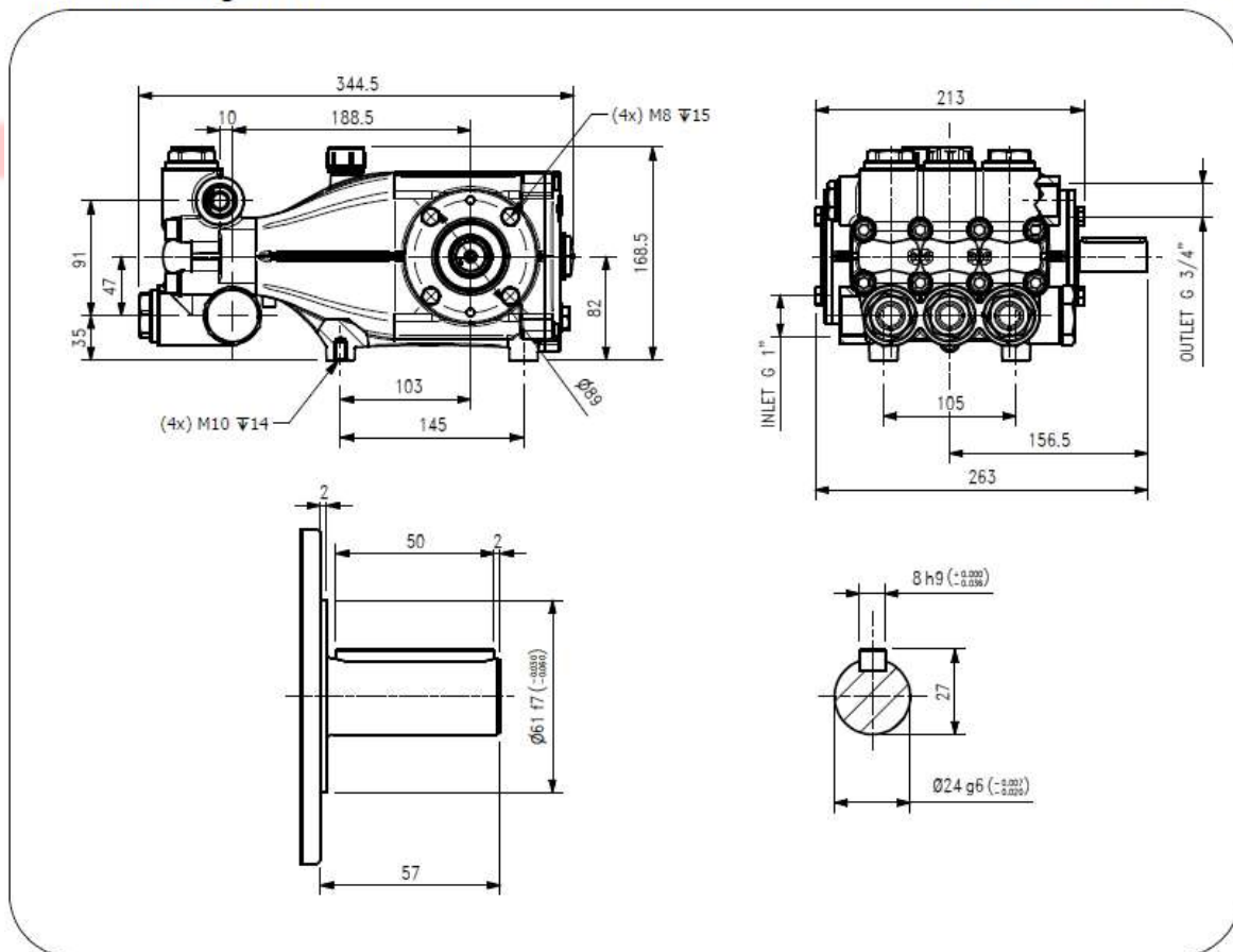
Dimensioni d'ingombro
